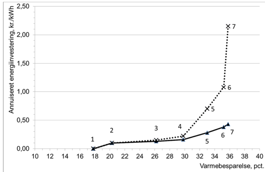
Figur 1 Annueret energiinvestering i kr./kWh i afhængighed af varmebesparelsen i pct. Optrukket kurve er summeret investering for scenarierne og stiplede kurve er marginal investering for det sidste scenarie. Tal på kurve er scenarienummer.
